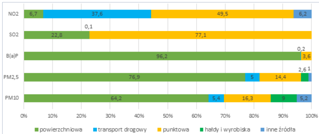
Wykres 18. Udziały źródeł w emisji zanieczyszczeń powietrza w województwie śląskim w 2019 r. (%)
