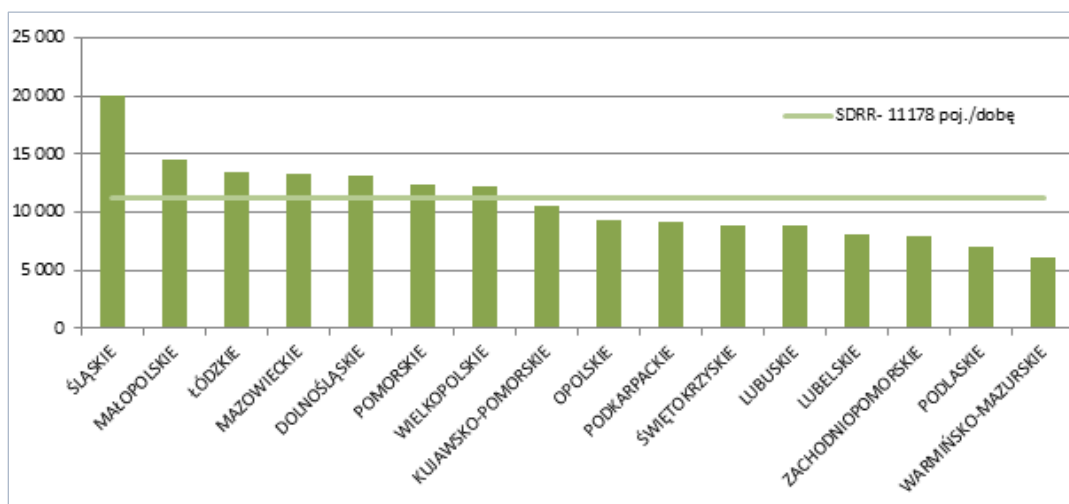
Wykres 19. Średni dobowy ruch roczny (SDRR) pojazdów silnikowych na sieci dróg krajowych w Polsce i województwach w 2015 r.
